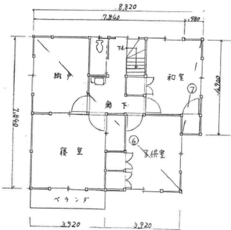
2F平面図 1/100
