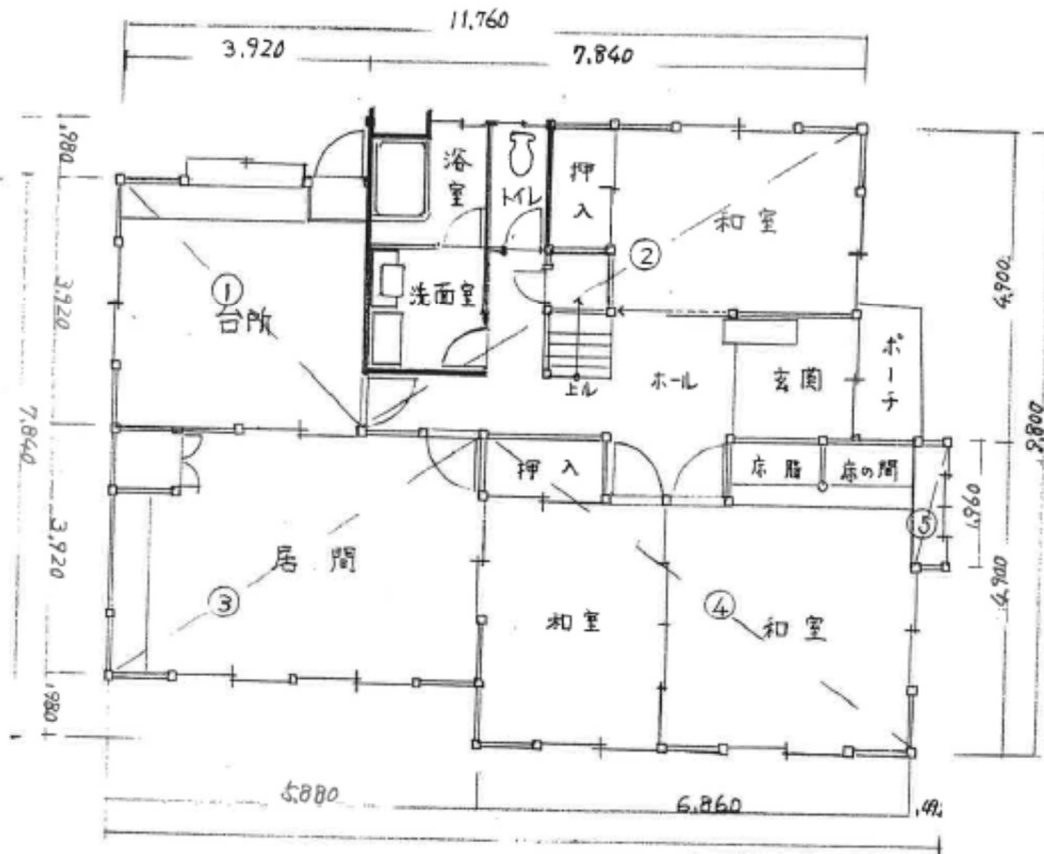
1F平面図 1/100
